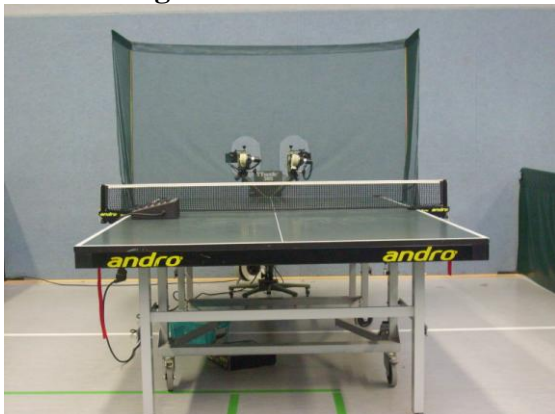
Anwendung eines Ballroboters
